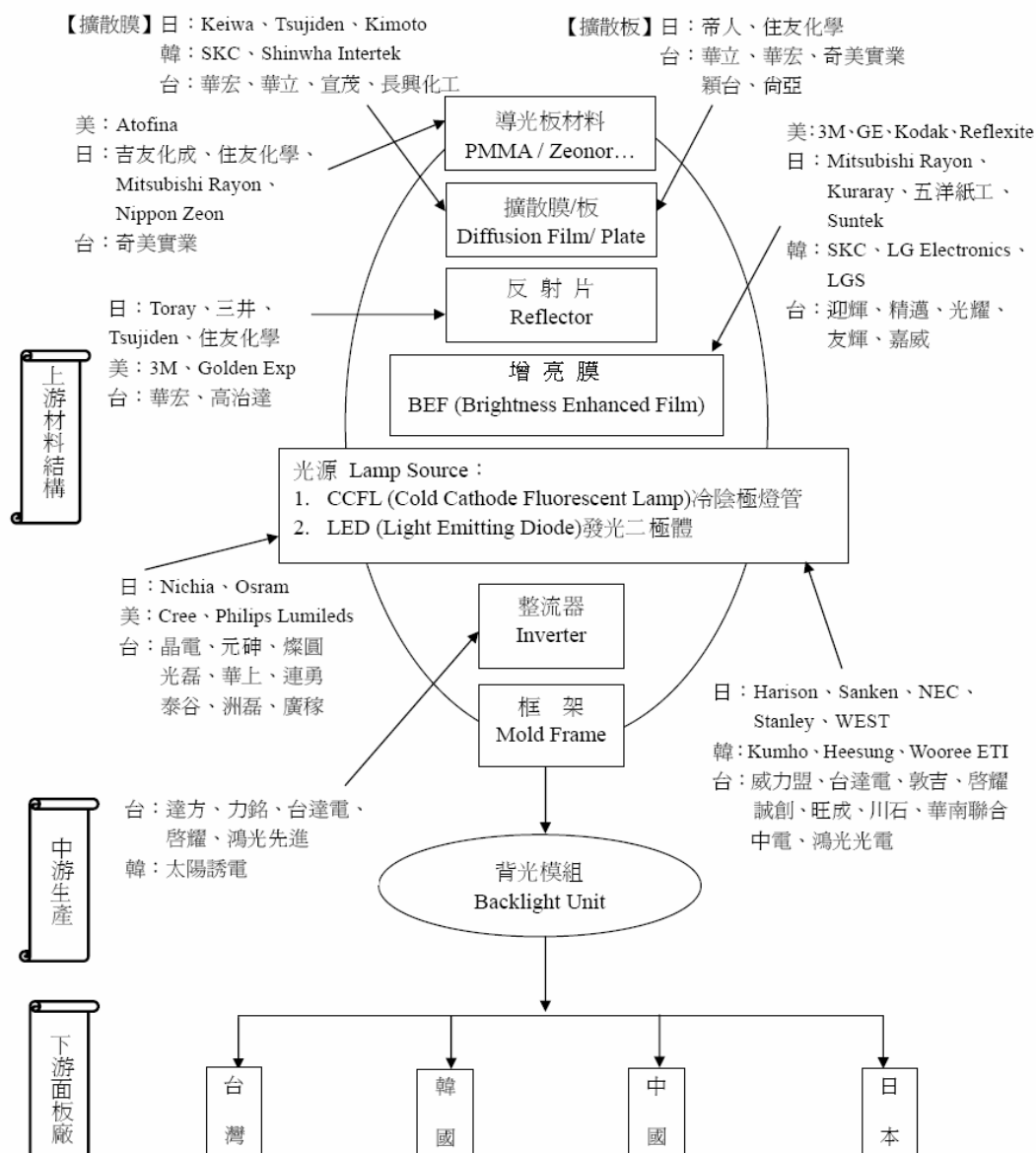
圖二、背光模組上、中、下游關聯圖
